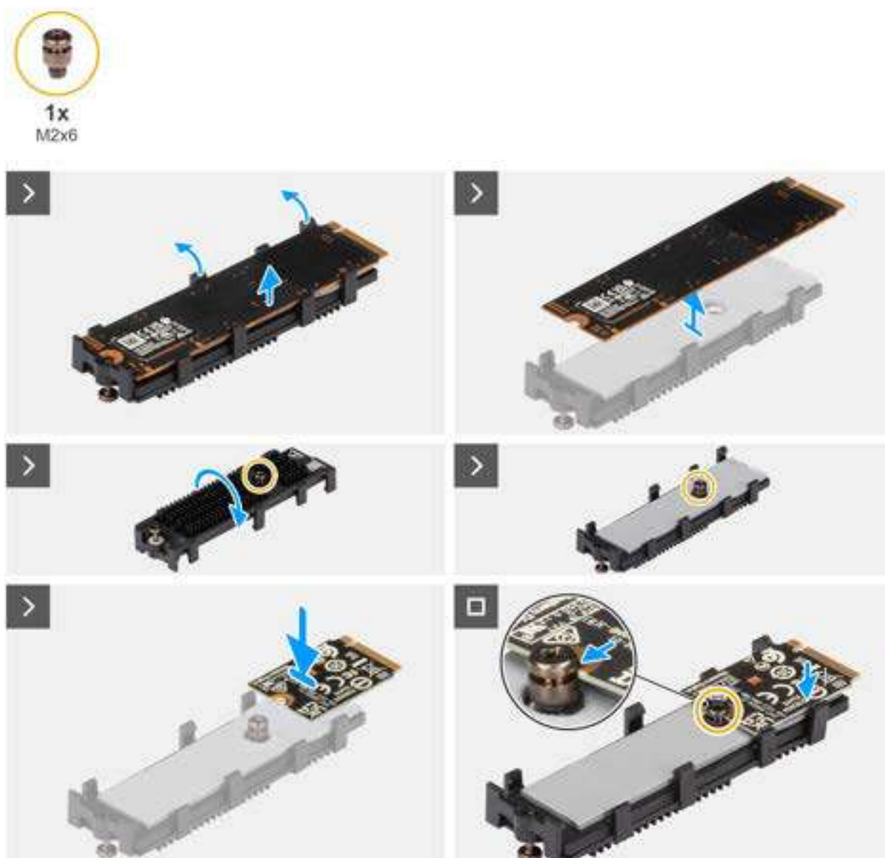
Figure 25. Remplacement du disque SSD M.2 2280 par un disque SSD M.2 2230
