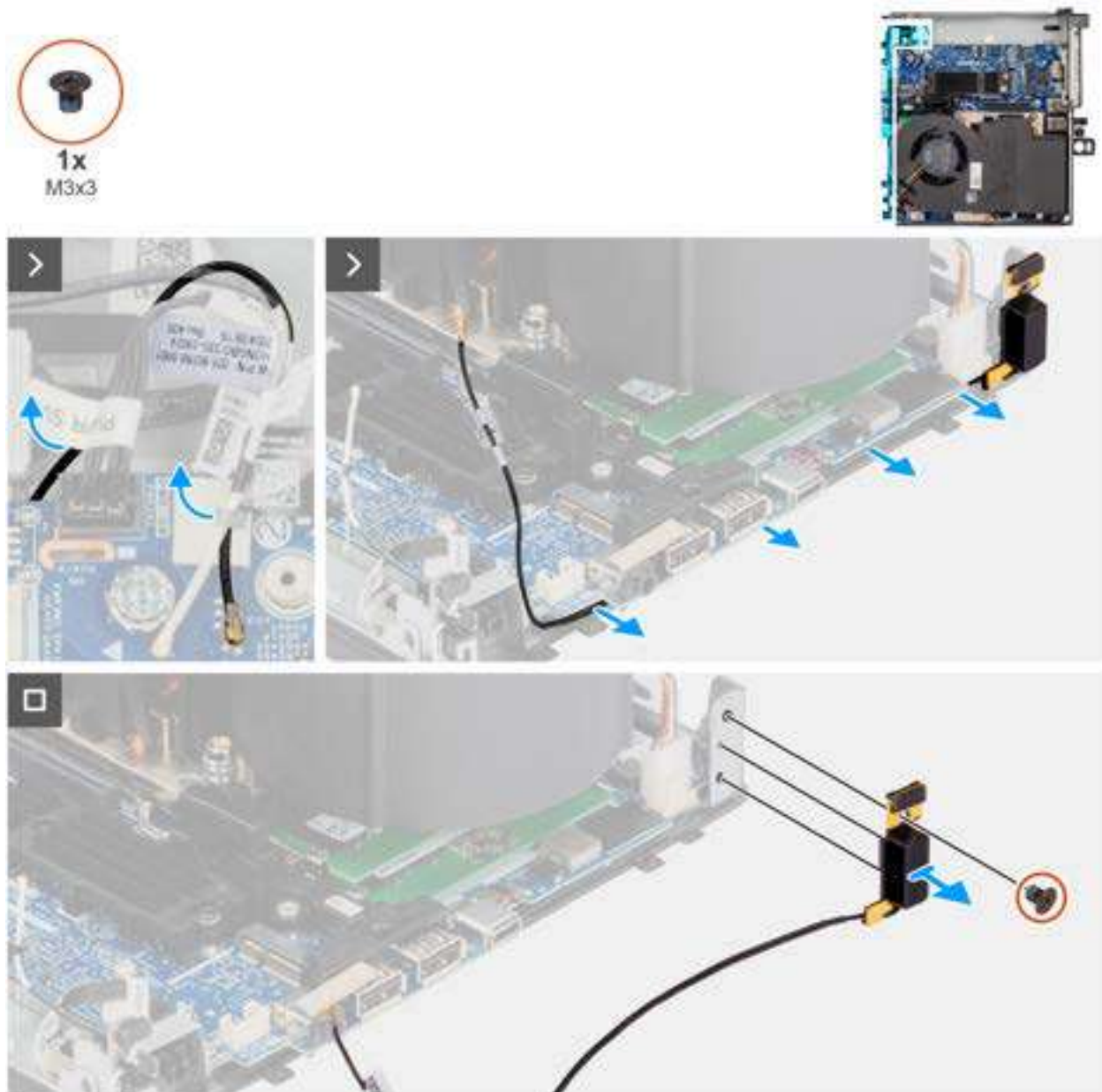
Figure 61. Retrait de l'antenne interne (emplacement 2)
