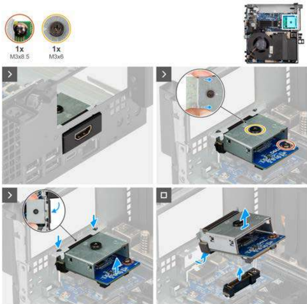
Figure 46. Retrait du port HDMI
