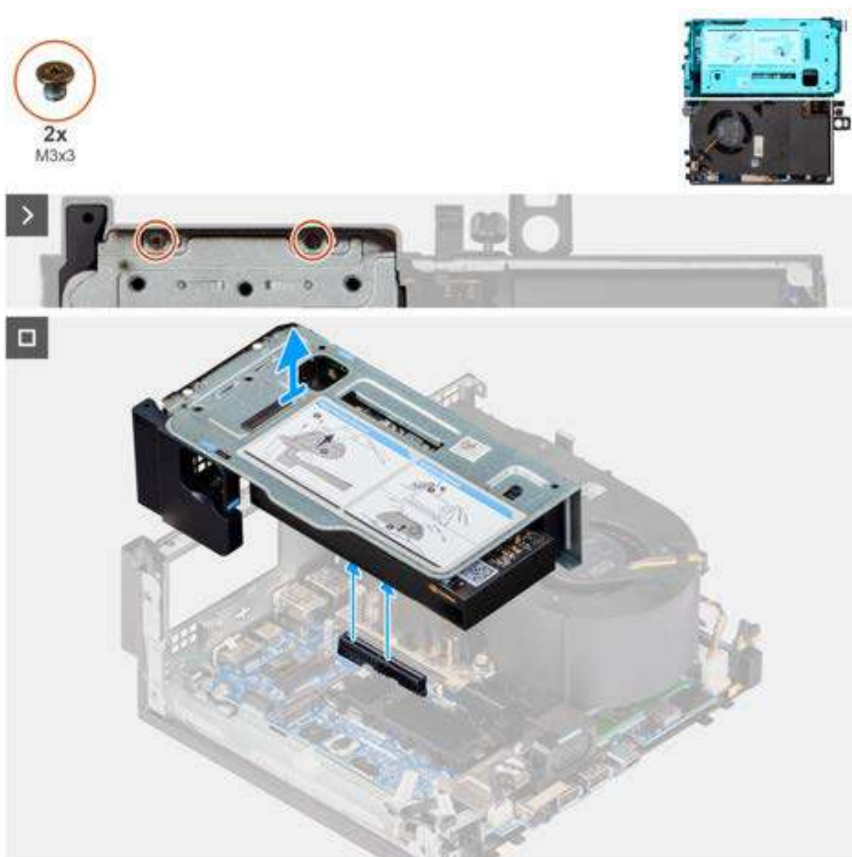
Figure 10. Retrait du module de la carte de montage
