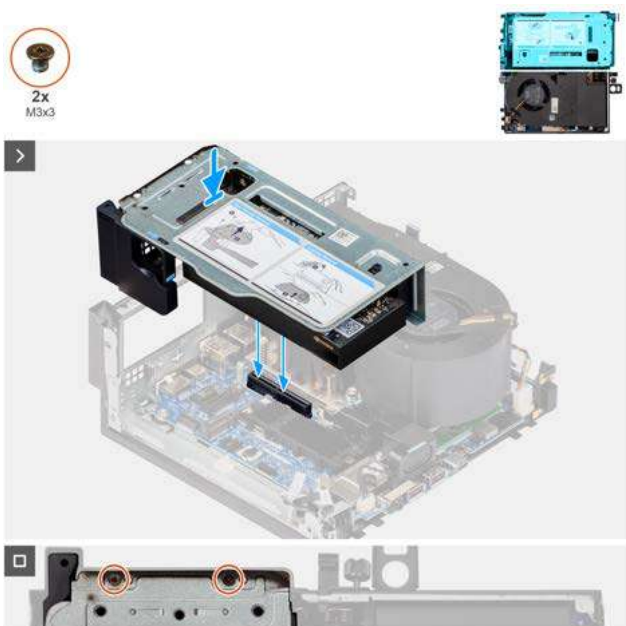
Figure 11. Installation du module de la carte de montage
