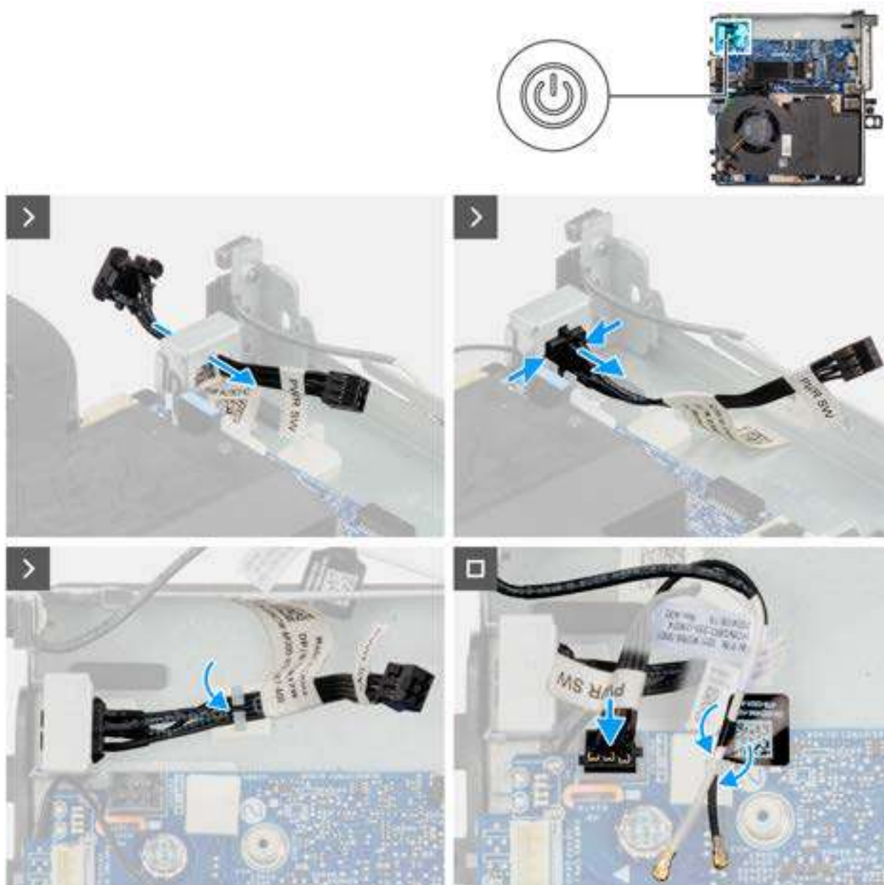
Figure 58. Installation du bouton d'alimentation
