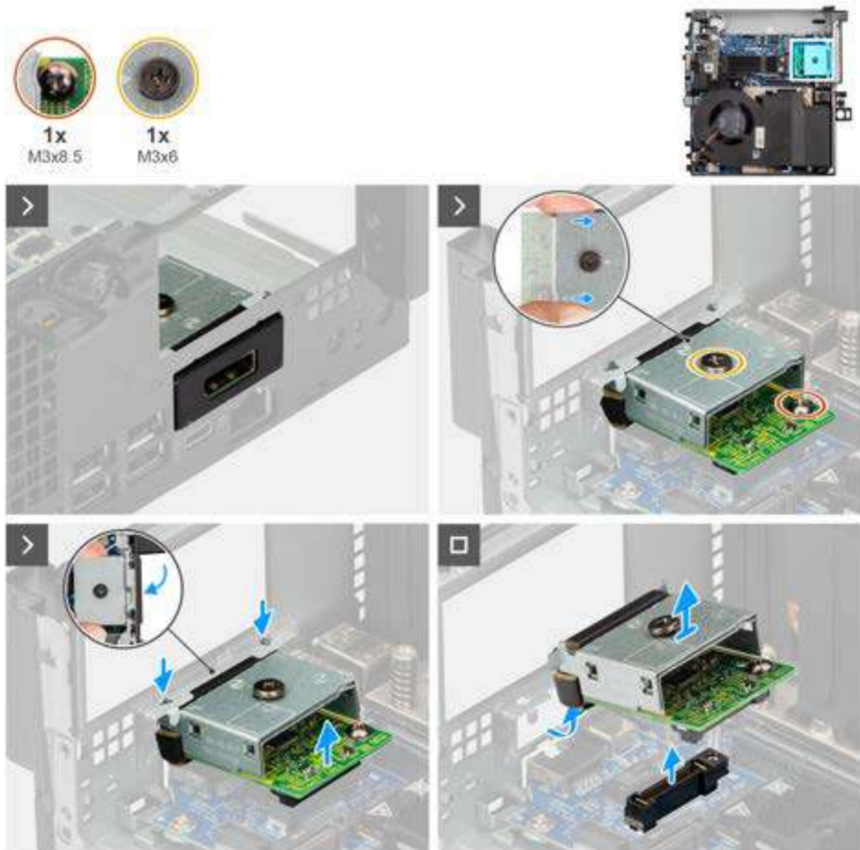
Figure 40. Retrait du port DisplayPort
