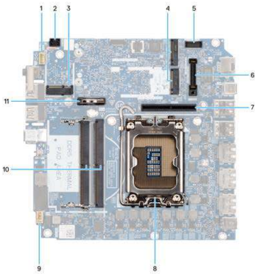
Figure 54. Connecteurs de la carte système
