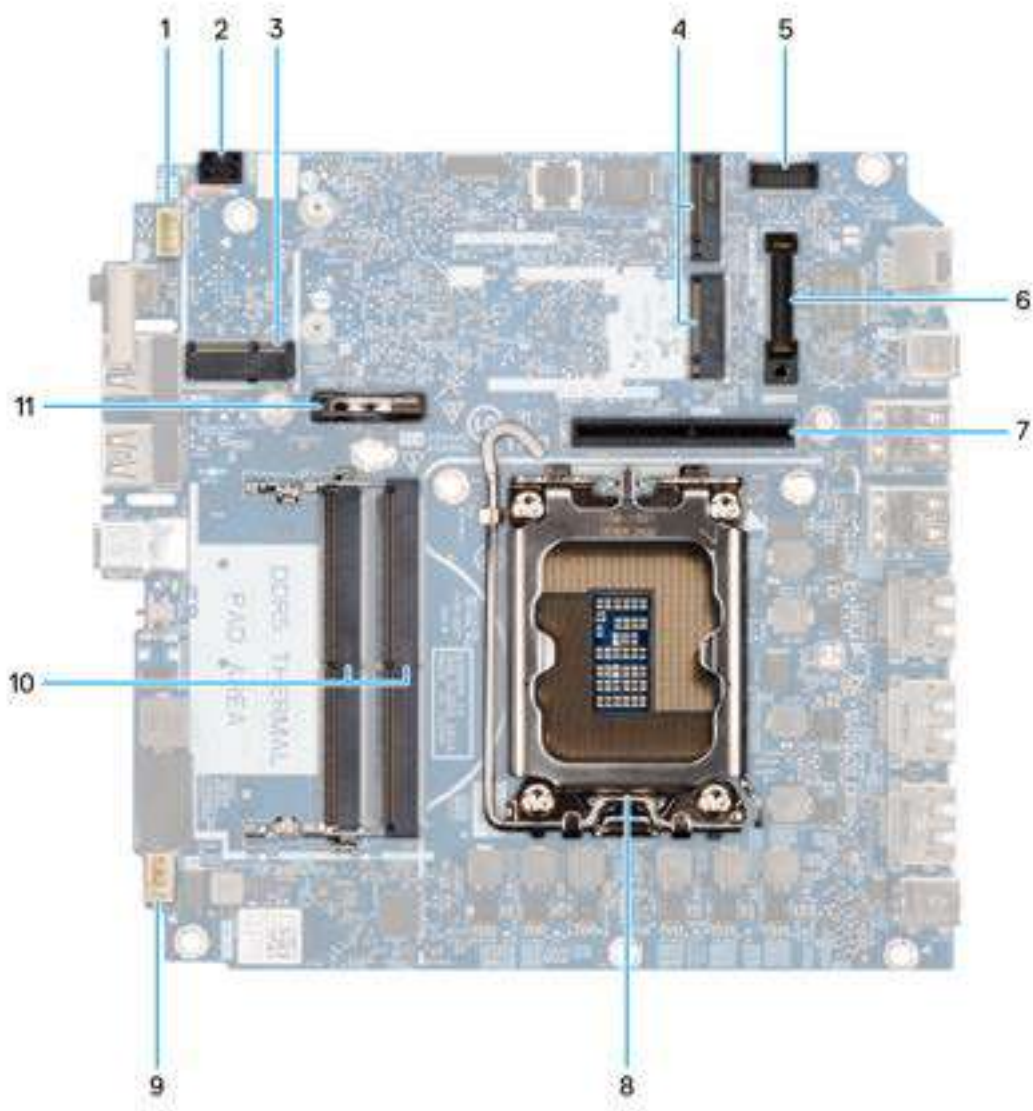
Figure 51. Connecteurs de la carte système
