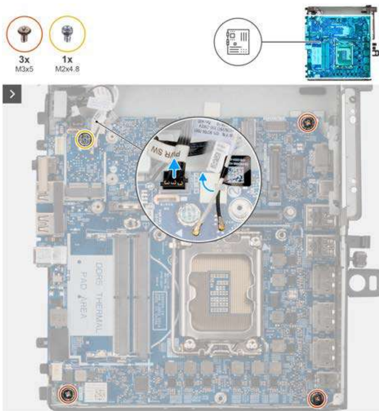
Figure 52. Retrait de la carte système
