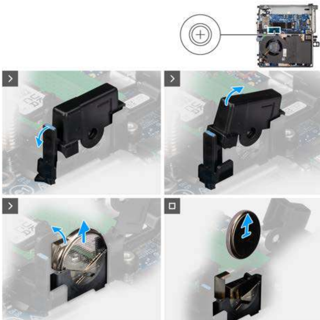
Figure 8. Retrait de la pile bouton
